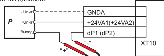
Датчик давления
