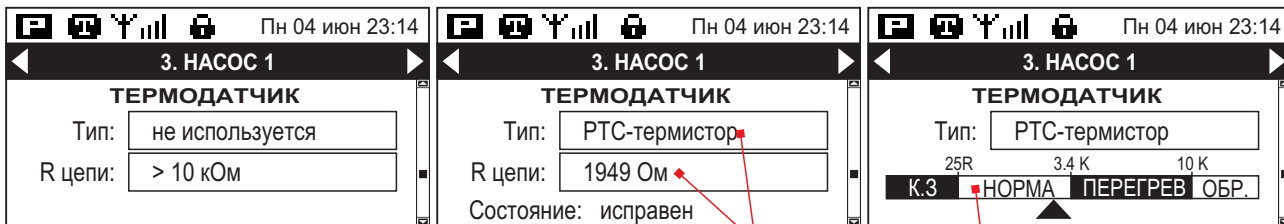
Тип термодатчика и его сопротивление Шкала состояния в зависимости от сопротивления Курсором указано текущее состояние
